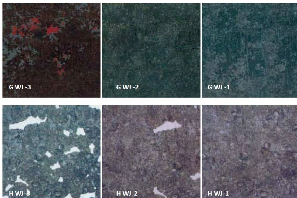
Figura 34 – Graus de corrosão
