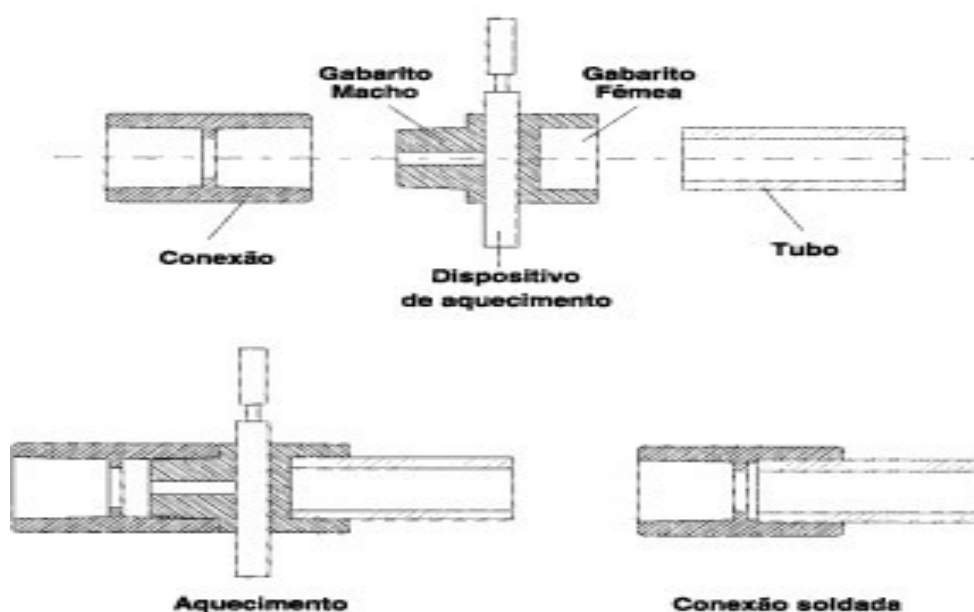
Figura 9 – Soldagem tipo soquete ou encaixe por termofusão
