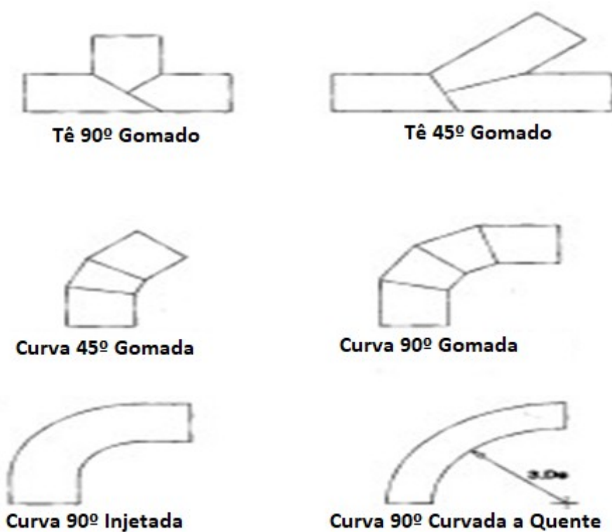
Figura 8 – Conexões para Solda de Topo por Termofusão 2
