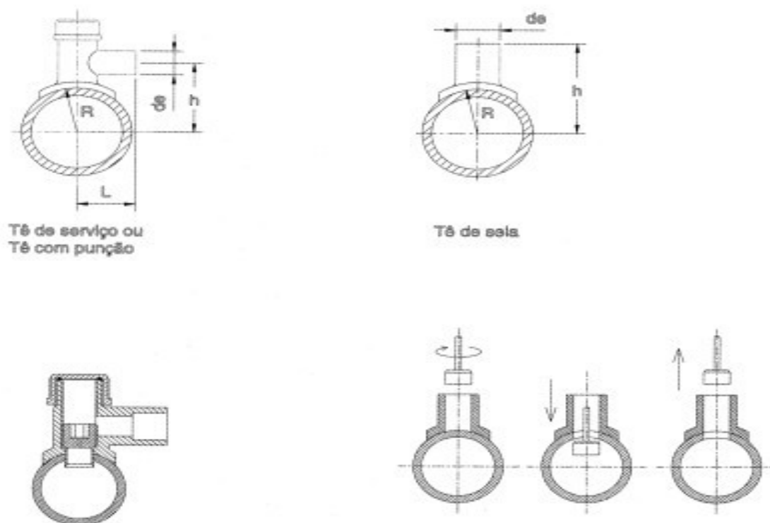
Figura 11 – Conexões para solda tipo Sela por Termofusão
