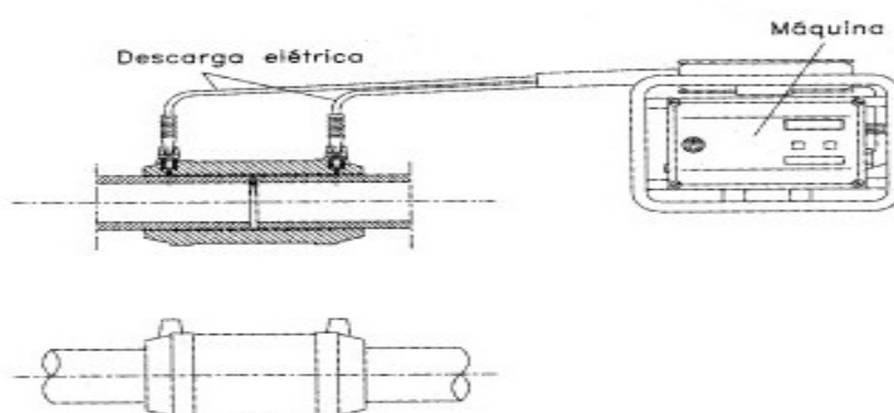
Figura 12 – Soldagem por eletrofusão
