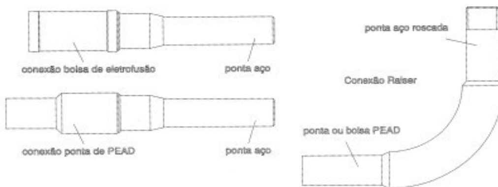
Figura 17 – Junta de Transição PE x Aço (Pontas)
