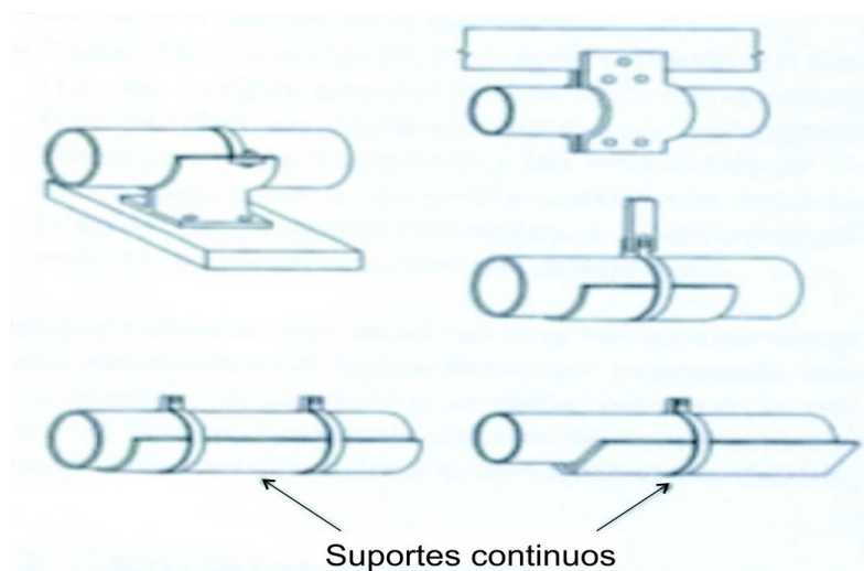
Figura 22 – Exemplos típicos de suportes de tubulações de HDPE
