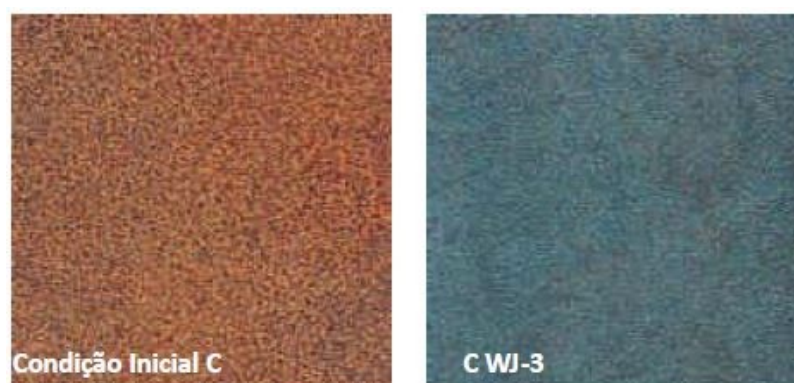
Figura 36 – Níveis de Flash Rust (C-WJ3)
