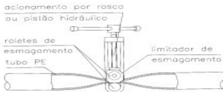
Figura 18 – Método do Estrangulador de Vazão (pinçador) O estrangulador deve ser qualificado.
