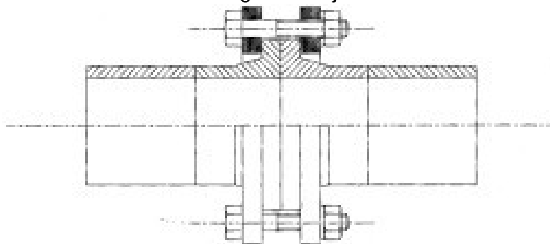
Figura 16 – Junta de Transição PE x Aço
