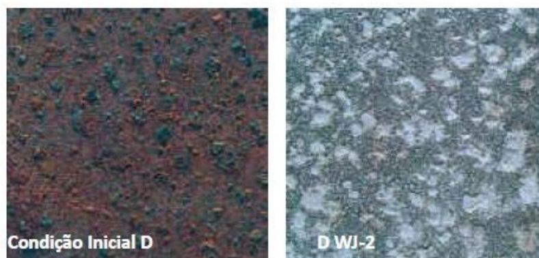
Figura 37 – Níveis de Flash Rust (D – WJ2)
