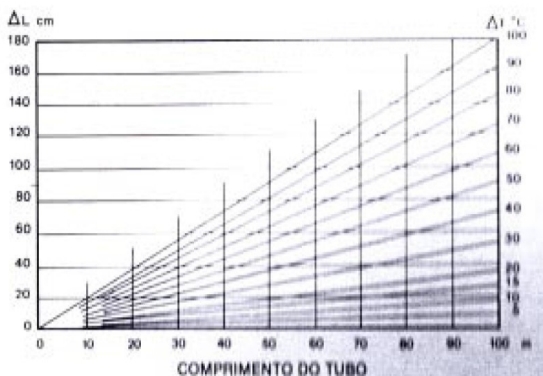
Figura 24 – Compensadores de dilatação - Efeito Lira
