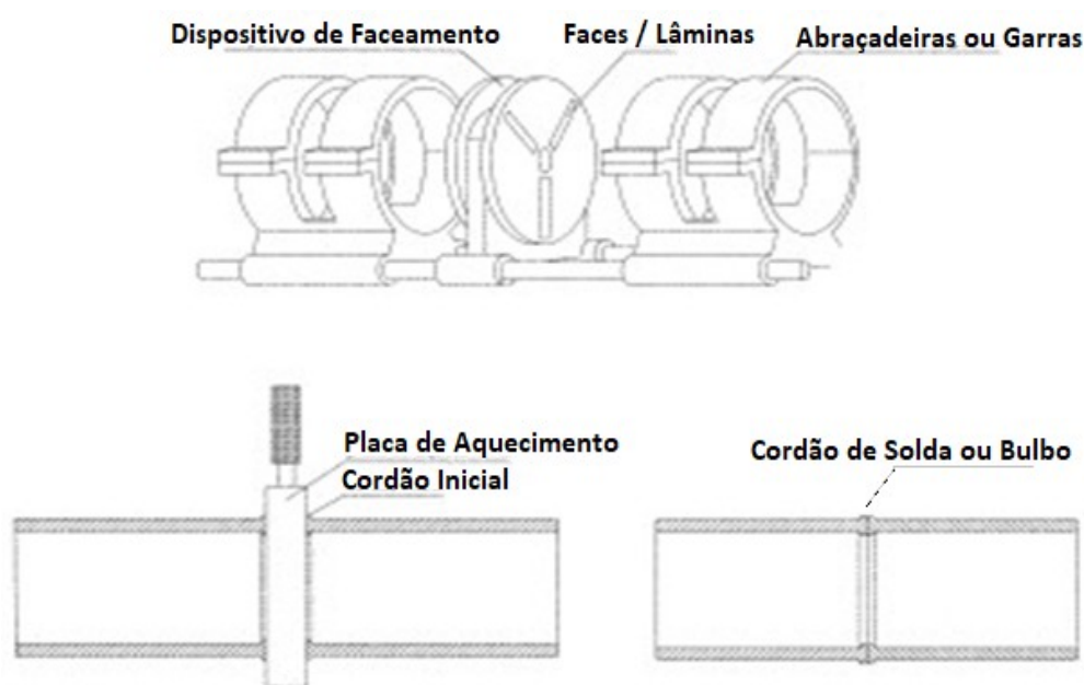
Figura 6 - Soldagem de topo por termofusao
