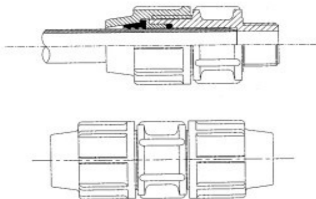
Figura 15 – Conexões de Eletrofusão
