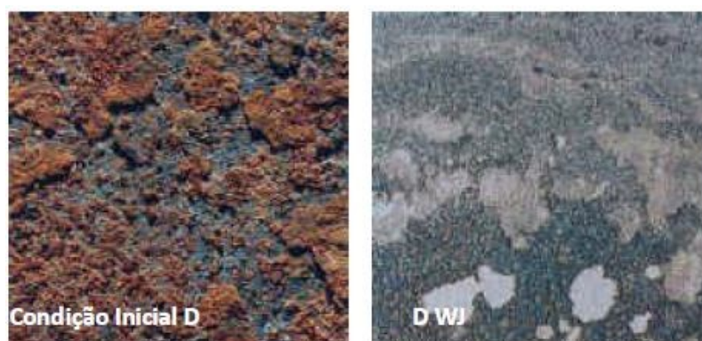
Figura 38 – Níveis de Flash Rust (D – WJ3)
