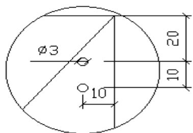
DETALHE DOS LACRES DIMENSÕES EM MILÍMETROS
