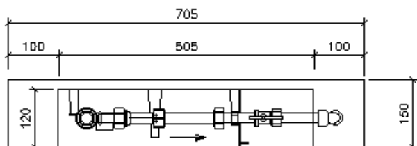
CORTE BB
