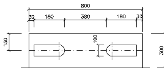
VISTA INFERIOR
