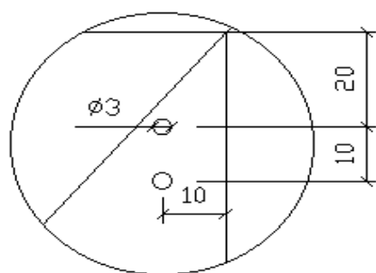
DETALHE DOS LACRES DIMENSÕES EM MILÍMETROS
