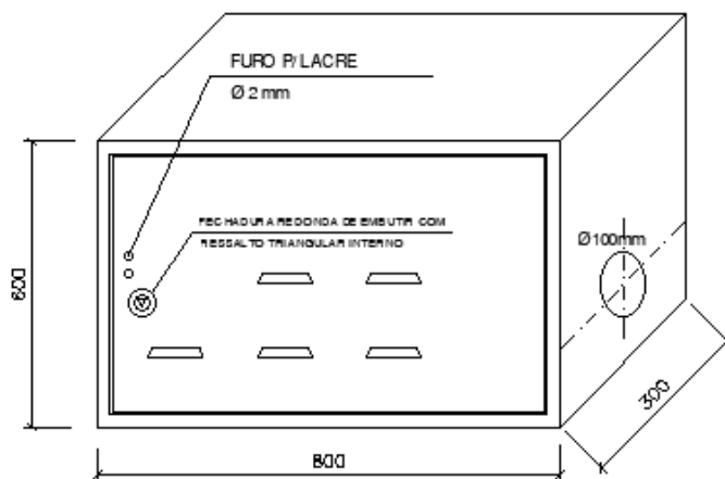
PERSPECTIVA
