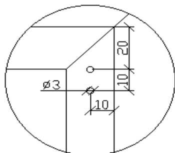
DETALHE DOS LACRES DIMENSÕES EM MILÍMETROS
