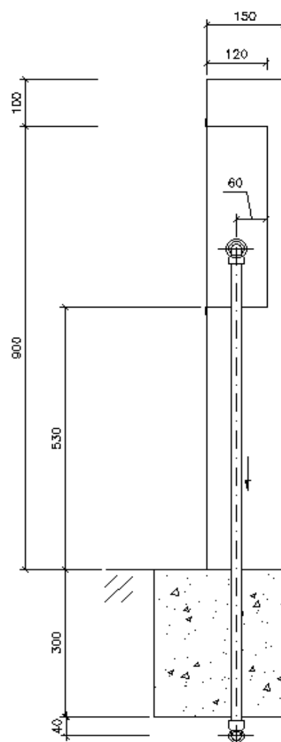
CORTE AA
