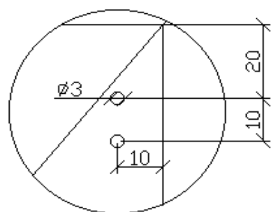
DETALHE DOS LACRES DIMENSÕES EM MILÍMETROS
