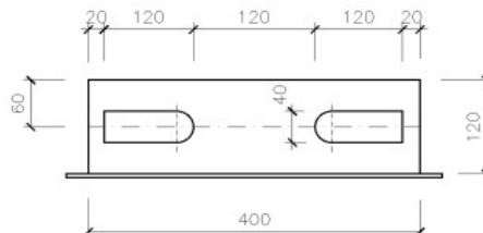
VISTA INFERIOR
