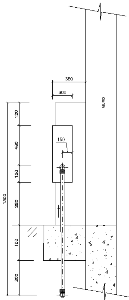
CORTE AA
