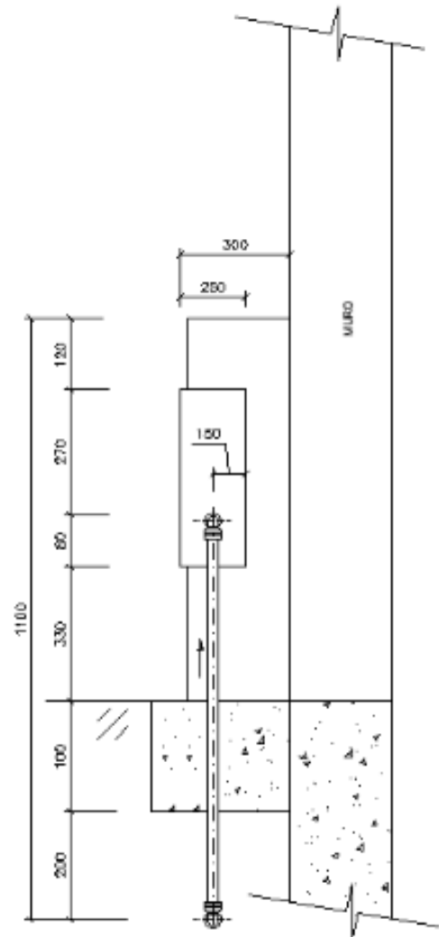
CORTE AA
