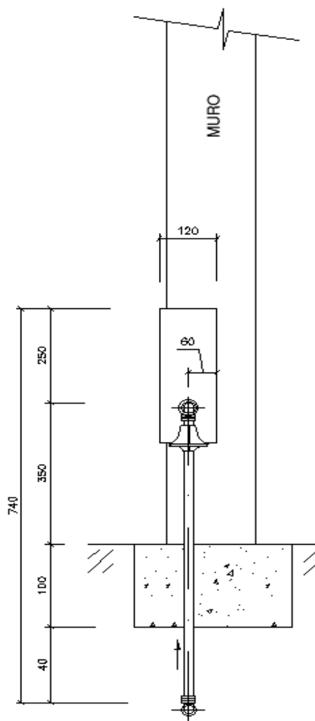
CORTE AA
