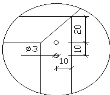
DETALHE DOS LACRES DIMENSÕES EM MILÍMETROS
