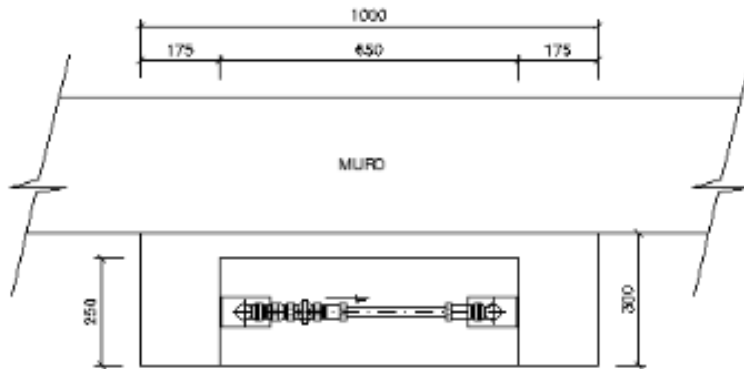
CORTE BB
