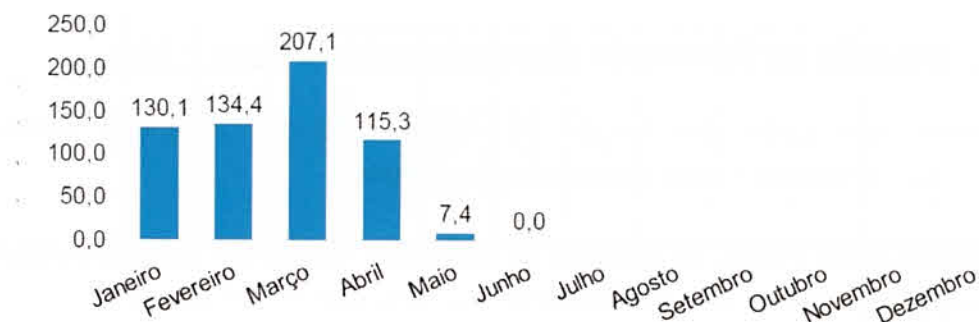
Gráficos 01 a 04 – Precipitação Acumulada 2015-2018 – Estação Barragem Ribeirão João Leite
