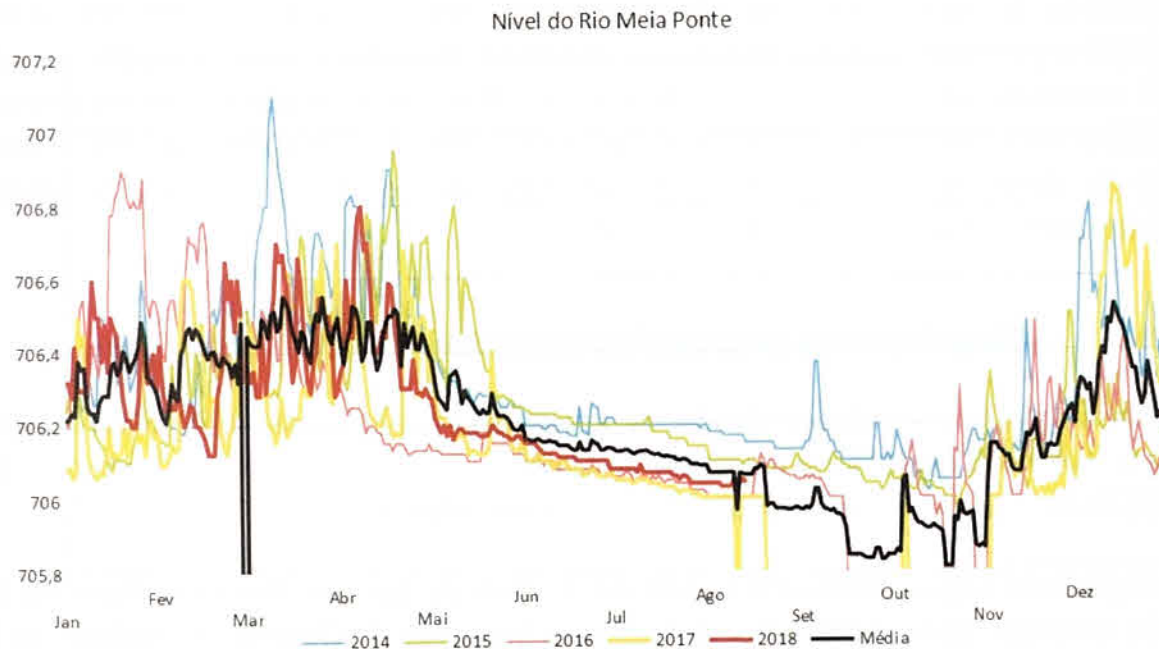
Gráfico 06 – Vazão Rio Meia Ponte – Ponto de Captação SANEAGO Goiânia – 2018
